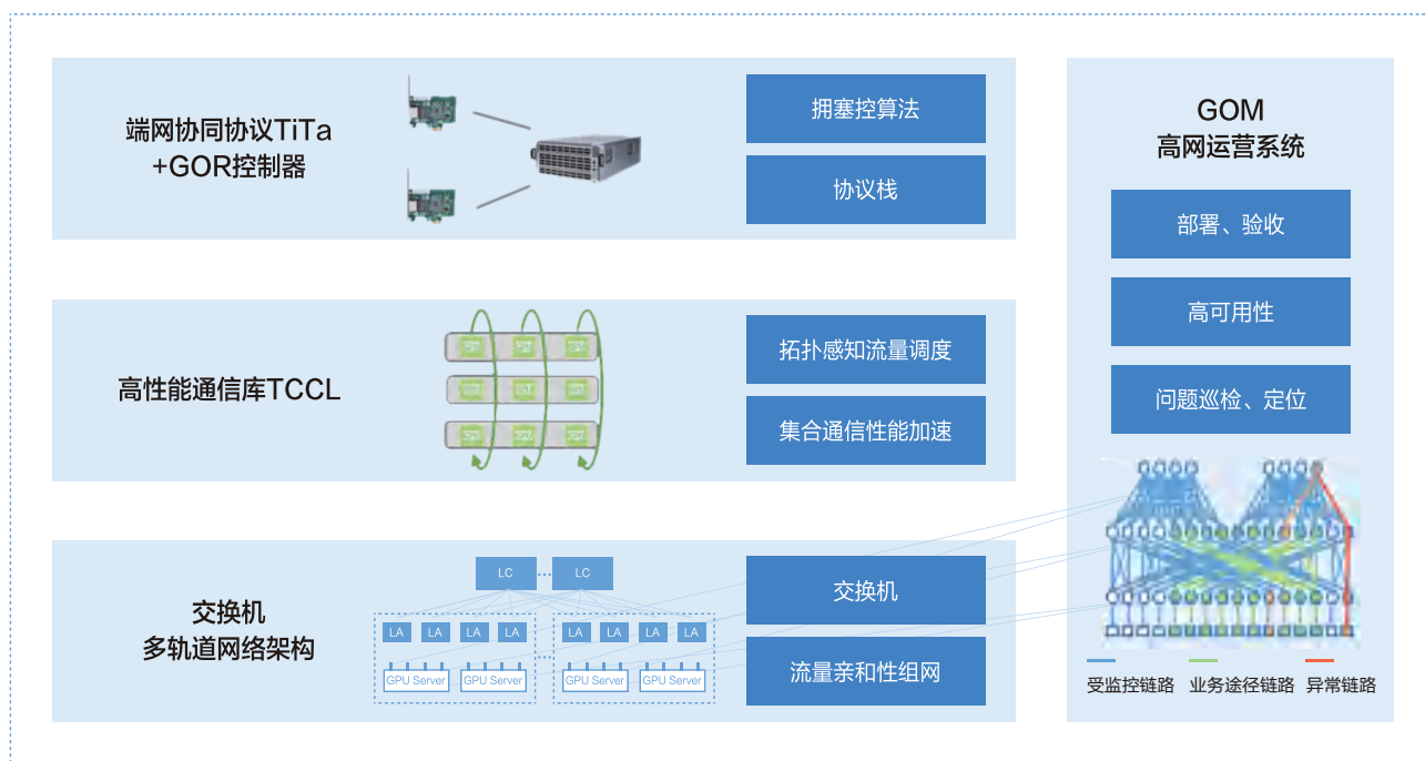
▲ 大模型训练新一代算力网络系统框架
