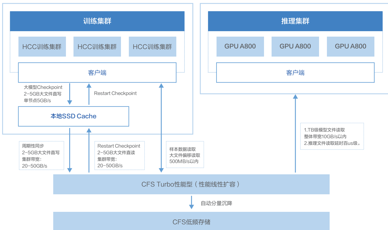
▲ CFS Turbo大模型解决方案
