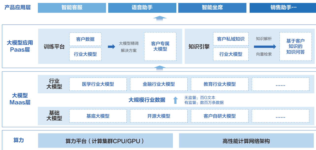
▲ 行业大模型框架
