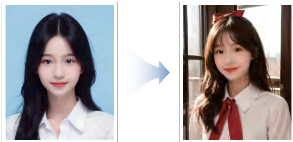
▲ AI写真
