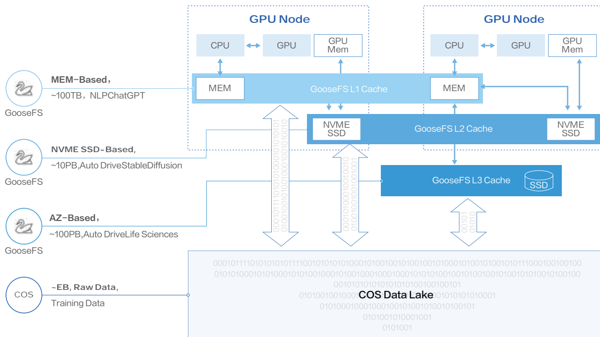
▲ COS+GooseFS缓存加速方案
