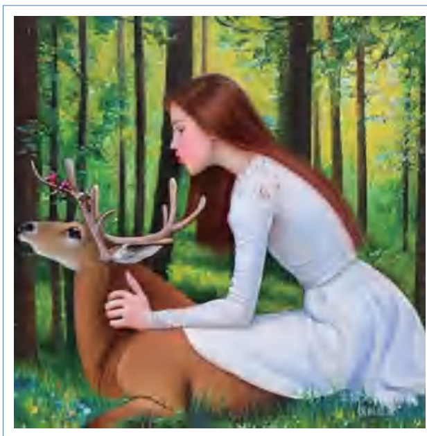
▲ 图片风格化
