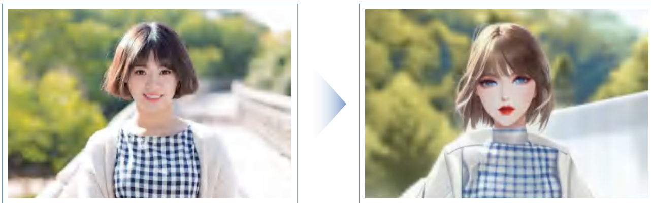
▲ 以图生图
